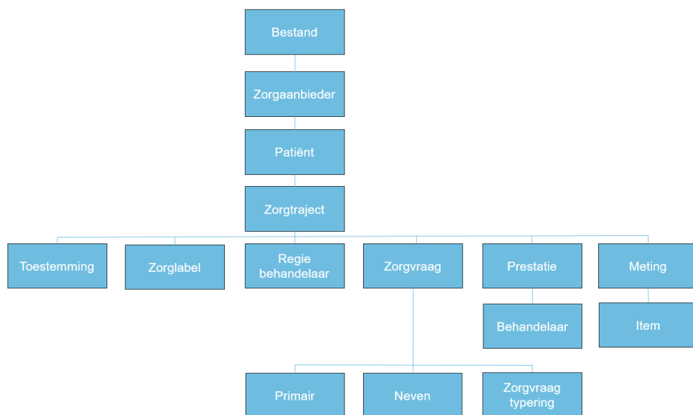
Figuur 1: Structuur van de dataset
